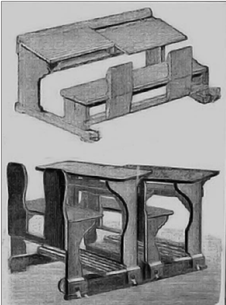
Модели Риккера, Кальмана, Дюрра
